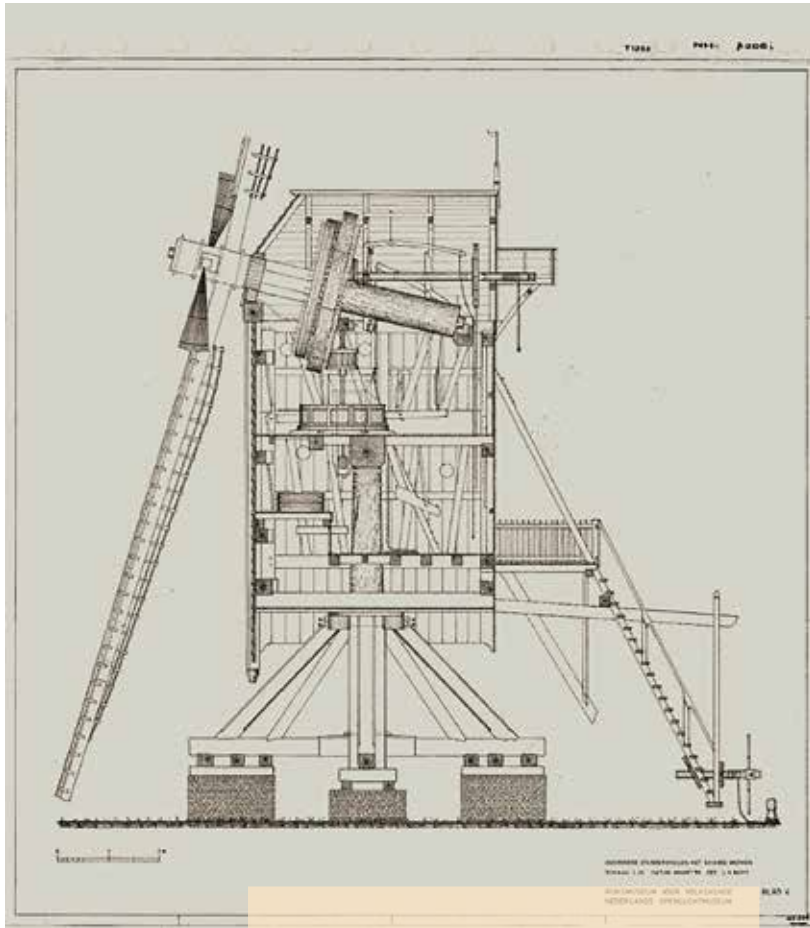
Een tekening van de doorsnede van de standerdmolen in het Openluchtmuseum te Arnhem. Deze molen stond oorspronkelijk in het Noord-Hollandse Huizen. De gehele constructie van de molen met de draaiende delen is hier getekend. (Tekening auteur 1986)
