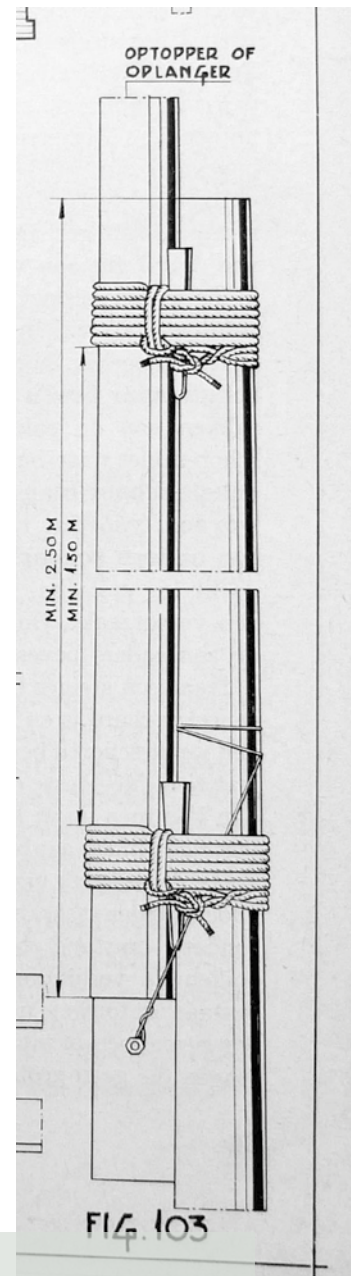
De in 1930 gebruikelijke verbindingen bij steigerwerk (R.Jellema, Gereedschappen, steigers en werktuigen in de bouw , 1963/64)
