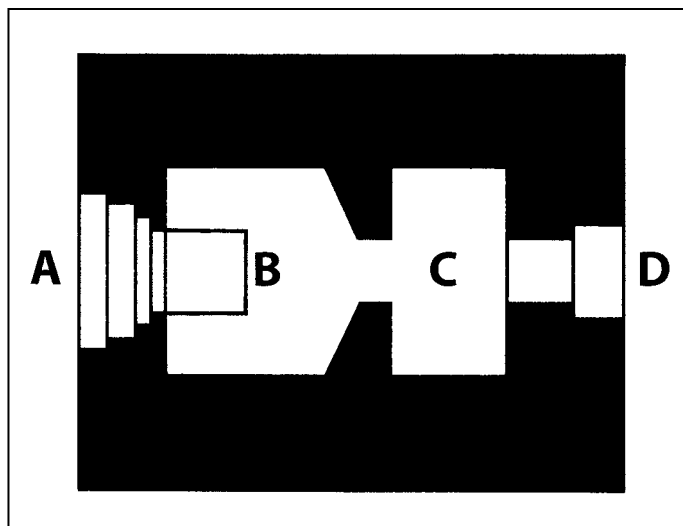
Plattegrond van de Regelbau 703 in De Klomp. L x b x h: 9,3 x 7,5 x 5,5 meter. A: Schietgat, B: Gevechtsruimte, C: Munitieruimte, D: Ingang (tekening G.M. Muller)
