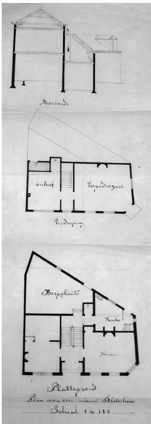
Bouwtekening van het tweede Polderhuis, 1900 (Gemeentearchief Veenendaal, Archiven gemeente Veenendaal 1811-1941, inv.nr. 279)
